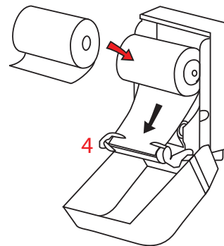
2-4 AUTOMATIC TRANSFER LOADING CHARGEMENT DE DISTRIBUTRICE Á TRANSFERT AUTOMATIQUE Carga de Transferencia Automàtica
