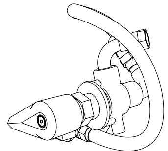
مقبض ذراع لصمام فردي (SVL)
