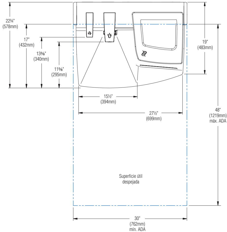
Vista superior
